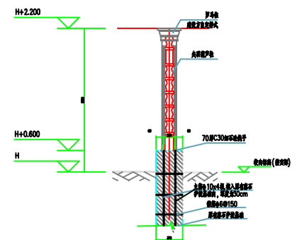
围墙做法剖面图
