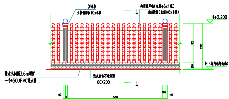
围墙做法正立面图
